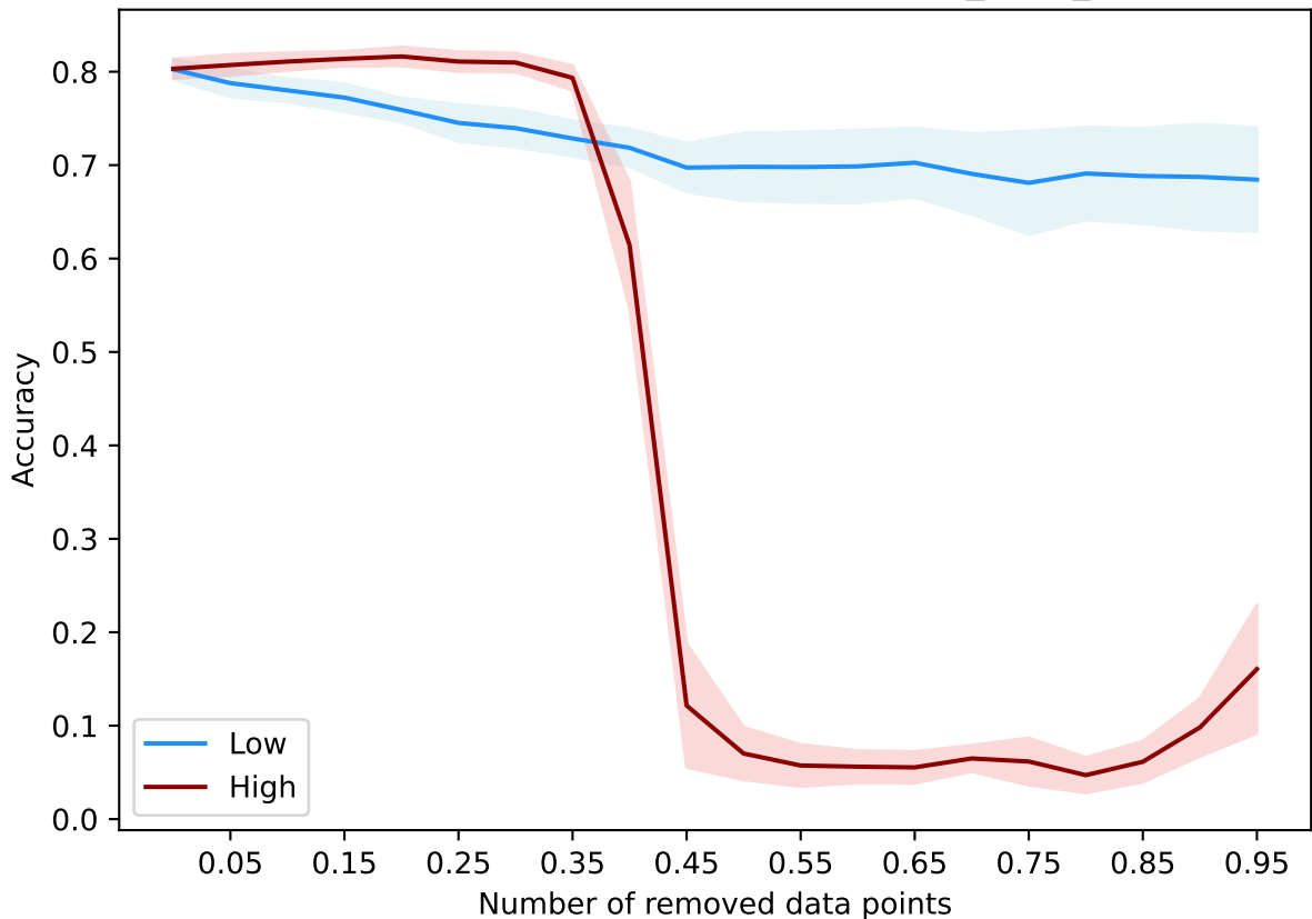
DataOob(1000, epochs=15) - polworst_class_acc
